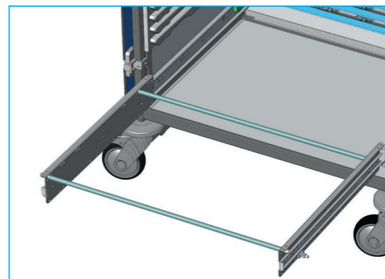
Cadres télescopiques pour une utilisation fixe de bacs dans le chariot
