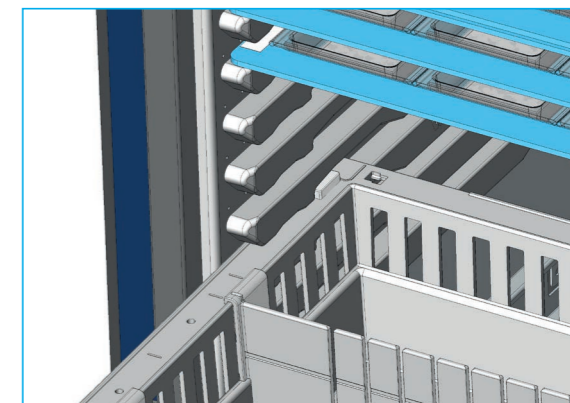
Les parois profilées permettent une utilisation plus flexible du chariot
