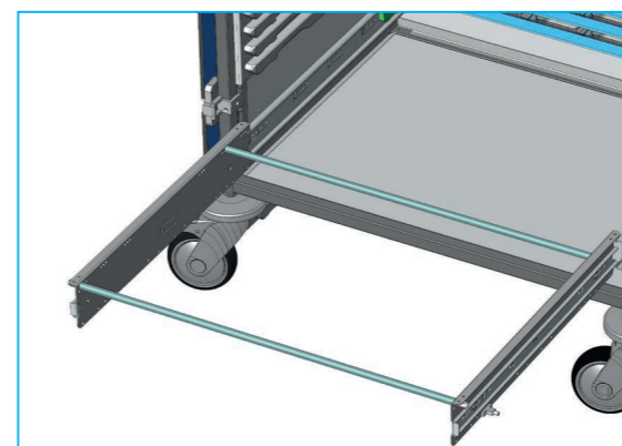
Telaio estraibile per l'utilizzo fisso di vasche nel carrello
