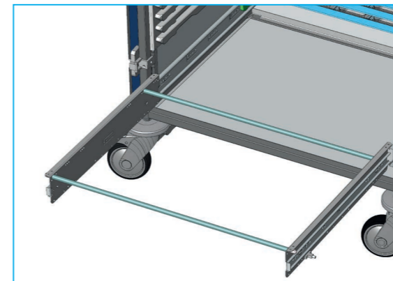
Auszugsrahmen für den fixen Einsatz von Modulen im Wagen
